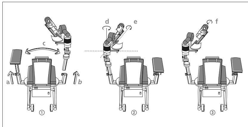
Esquema de conversión de ARTROMOT®-E2:
